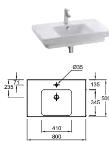
Vanity top L 80 x 50 cm E4796 - €432 incl. VAT
