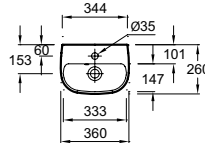
Handwash basin 36 x 26 cm E4761 - €119 incl. VAT
